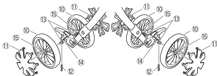
後車輪詳細図
